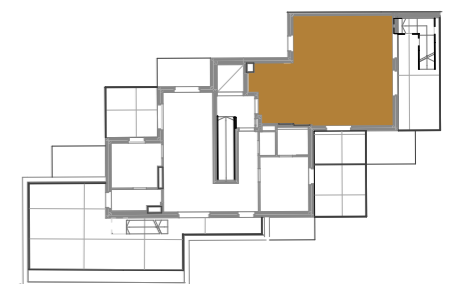
5. OG GESCHOSSPLAN
